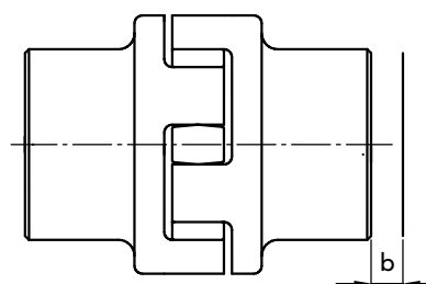
Disassamento ASSIALE
