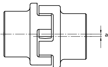
Disassamento RADIALE
