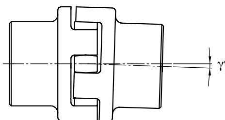
Disassamento ANGOLARE
